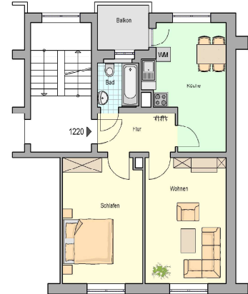
Raumbezeichnung beispielhaft
