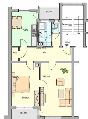
Raumbezeichnung beispielhaft
