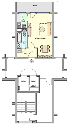
Raumbezeichnung beispielhaft
